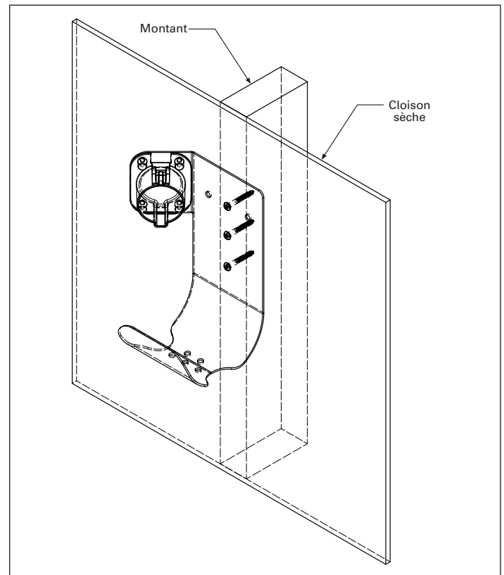
Figure 2. Fixer l'étui à cordon de qualité supérieure au mur
