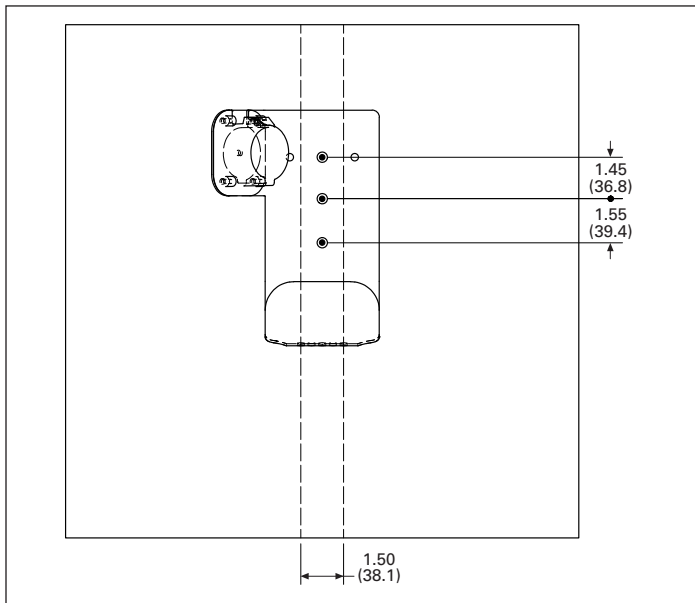
Figure 1. Dimensions des trous de montage en po (mm)
