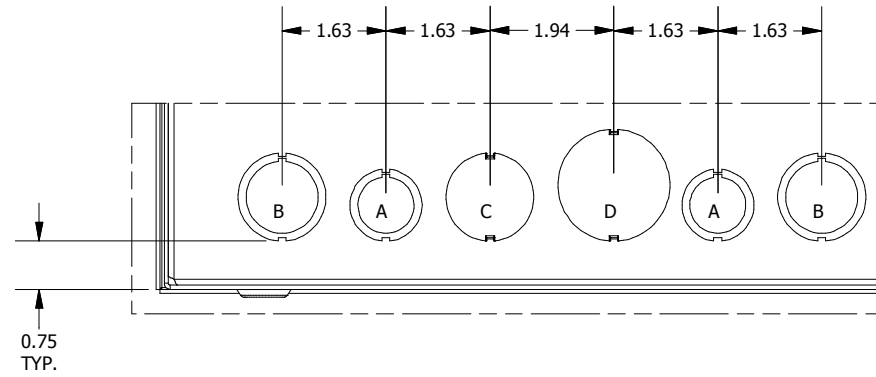
DETAIL B (2 PL.) (K.O. PATTERN)
