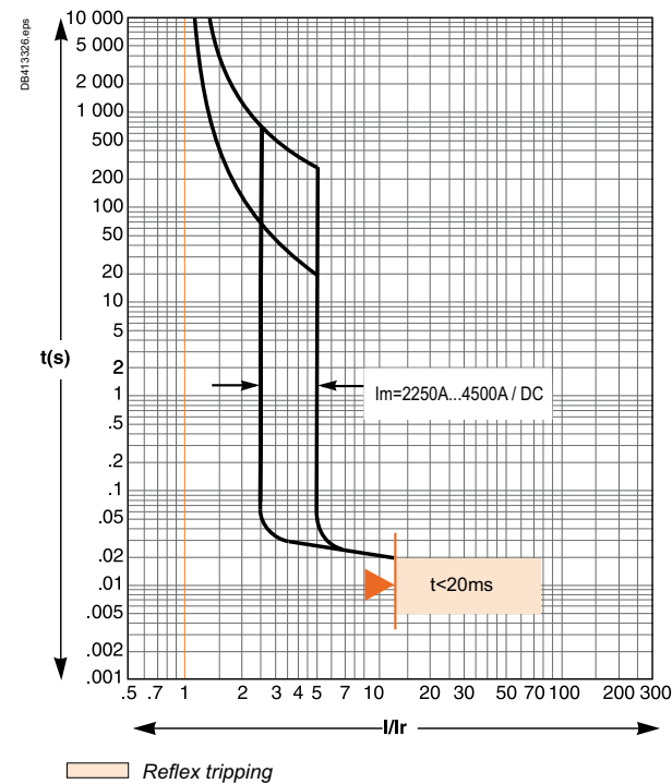
L-Frame 1200A
