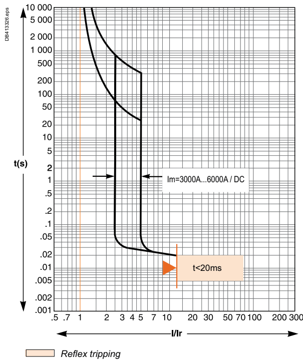
L-Frame 1200A
