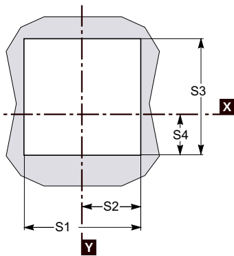
Front-Panel Cutout
