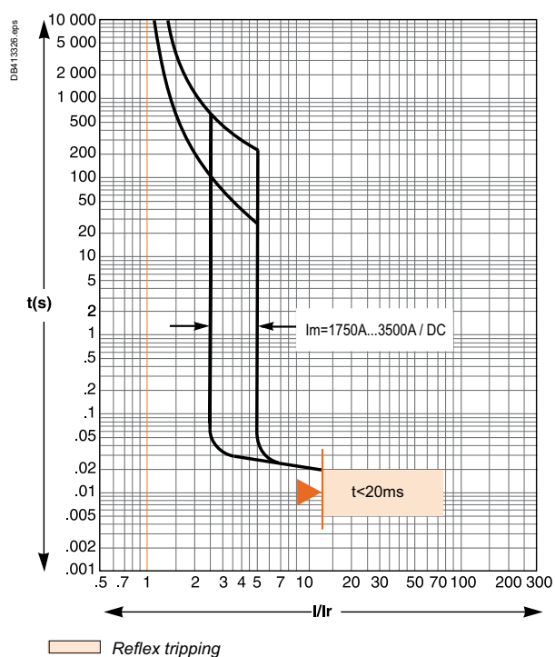
L-Frame 700A
