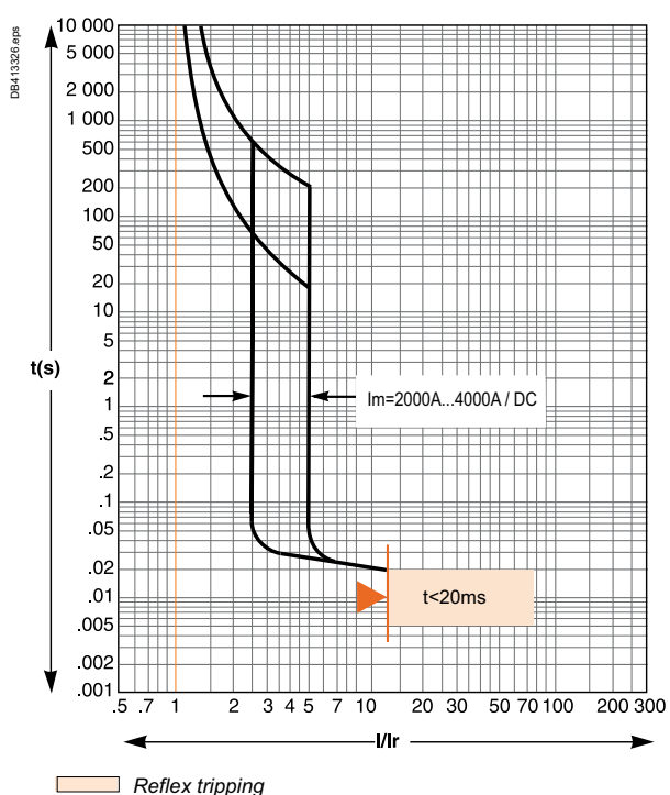
L-Frame 800A
