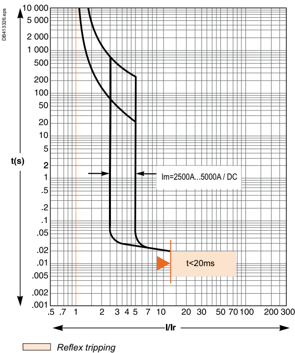
L-Frame 1000A
