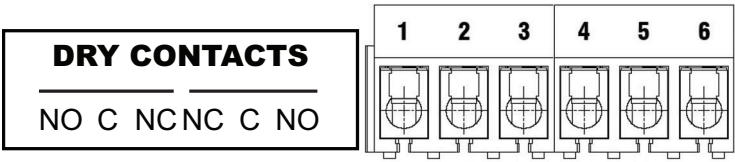
Figure 10 : Configuration de la carte des contacts secs
