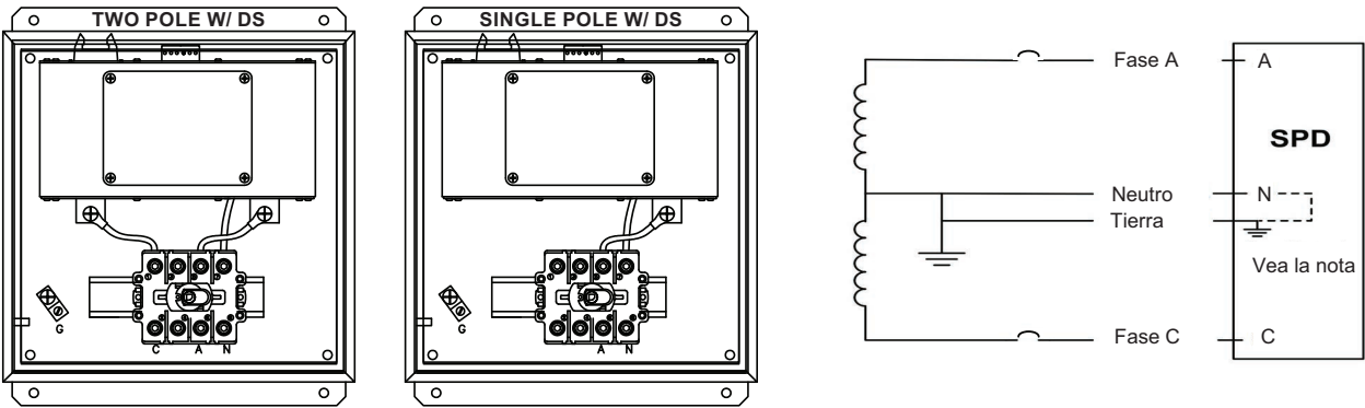
Figura 4: Instalación con conexión a tierra de una fase, tres hilos y desconectador integral
