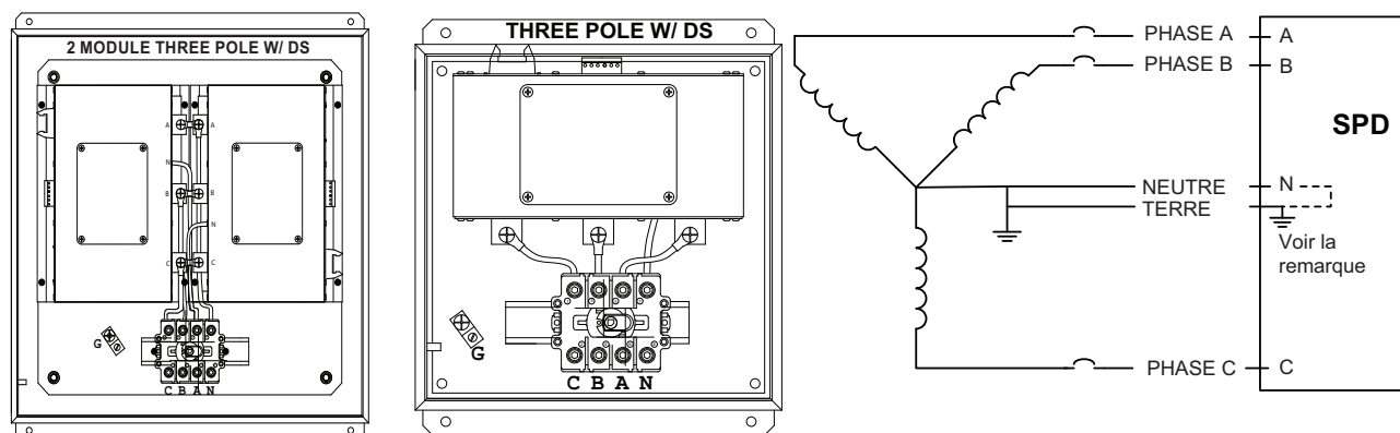
Figure 5 : Installation triphasée, à trois ou quatre fils, mise à la terre, en étoile avec commutateur intégré
