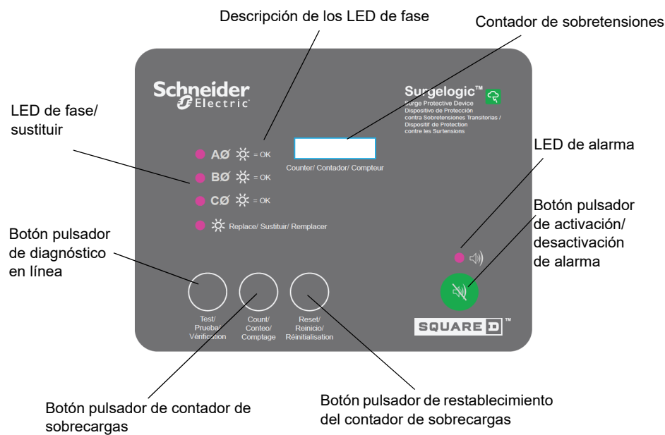
Figure 9: Panel de la pantalla de diagnóstico trifásico con contador de sobretensiones
