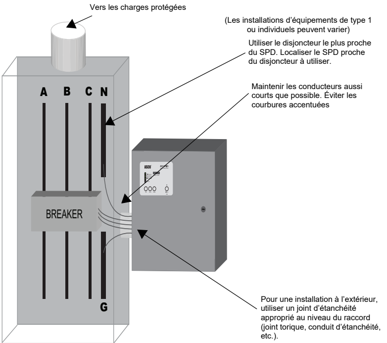
Figure 3 : Installation typique du panneau
