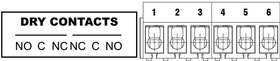
Figura 10: Configuración de los contactos secos
