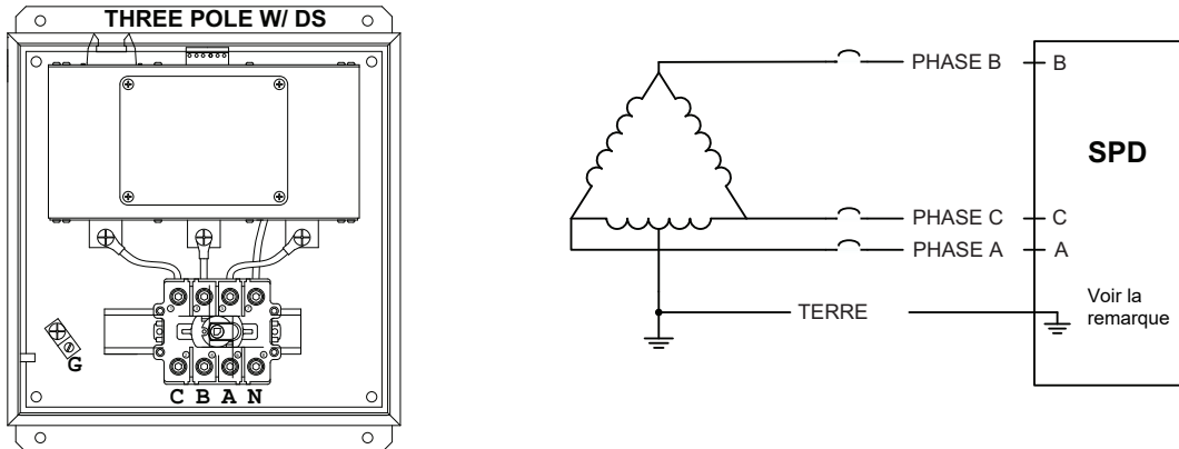
Figure 6 : Installation triphasée, 3 ou 4 fils, en sommet de triangle avec commutateur intégré
