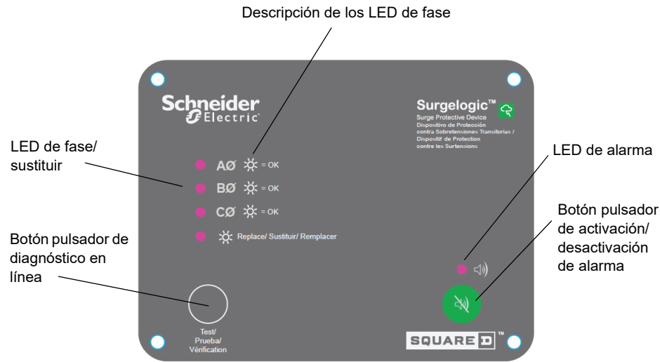
Figura 8: Pantalla de diagnóstico de tres fases con contador de sobretensiones transitorias
