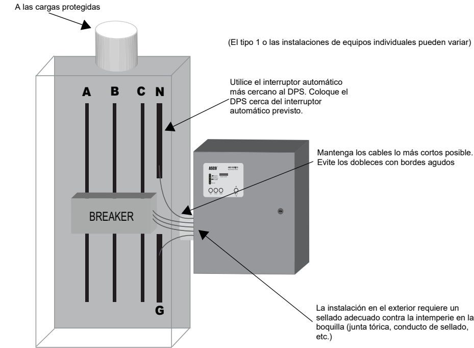
Figura 3: Instalación típica del tablero
