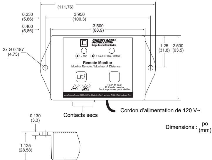
Figure 12 : Option de moniteur à distance (TVS12RMU)
