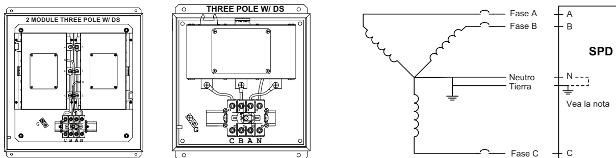
Figura 5: Instalación en estrella con conexión a tierra de tres fases, 3 o 4 hilos y desconectador integral
