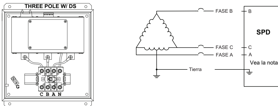
Figura 6: Instalación en delta con extremo alto de 3 fases, 3 o 4 hilos con desconectador integral
