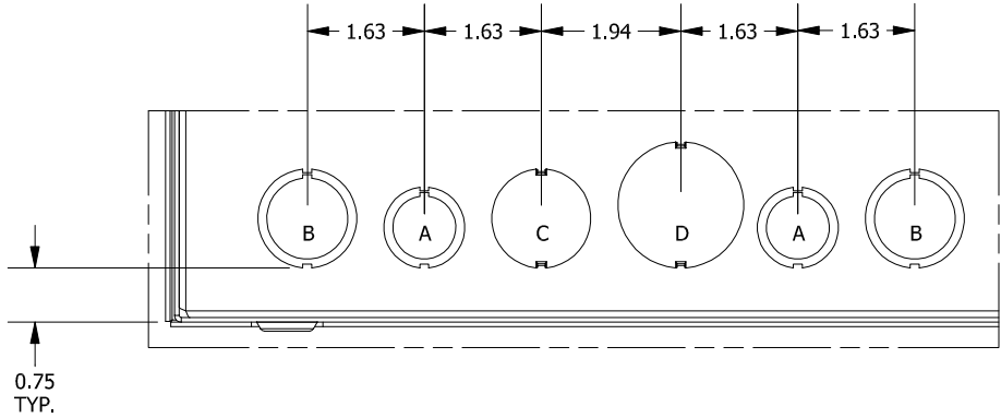
DETAIL B (2 PL.) (K.O. PATTERN)
