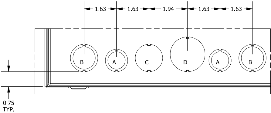
DETAIL B (4 PL.) (K.O. PATTERN)
