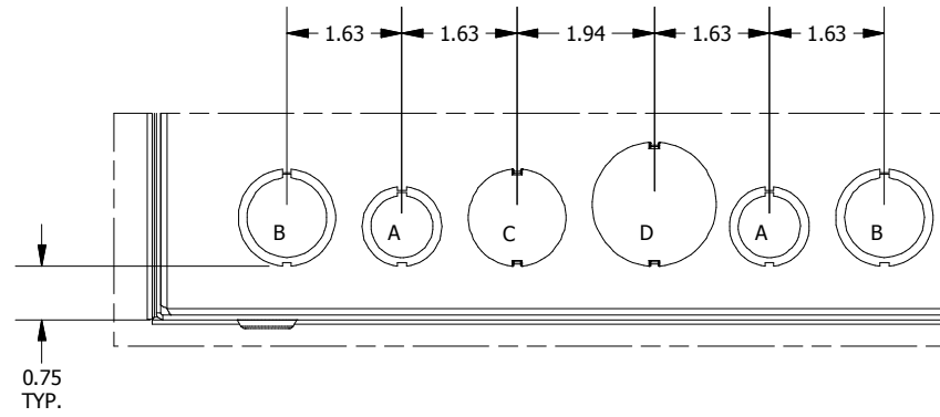
DETAIL B (3 PL.) (K.O. PATTERN)
