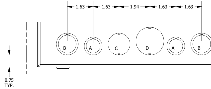
DETAIL B (5 PL.) (K.O. PATTERN)
