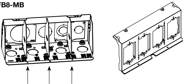
EFB8-MB
