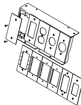
10 Gang Plate layout Disposition de la plaque simple 10 10 Plantillas de placa de salida
