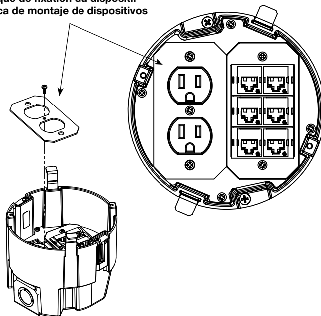
Device Mounting Plate Plaque de fixation du dispositif Placa de montaje de dispositivos
