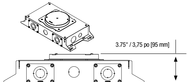
RFBA2C30 & RFBA2C30OG with collar / avec collier / con collarín
